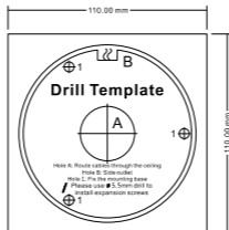
Рисунок 2-2 Шаблон крепления
