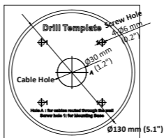
Рисунок 2-7 Шаблон крепления
