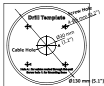
Рисунок 2-10 Шаблон крепления
